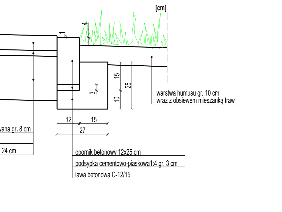
Szczegół krawędzi zjazdu
