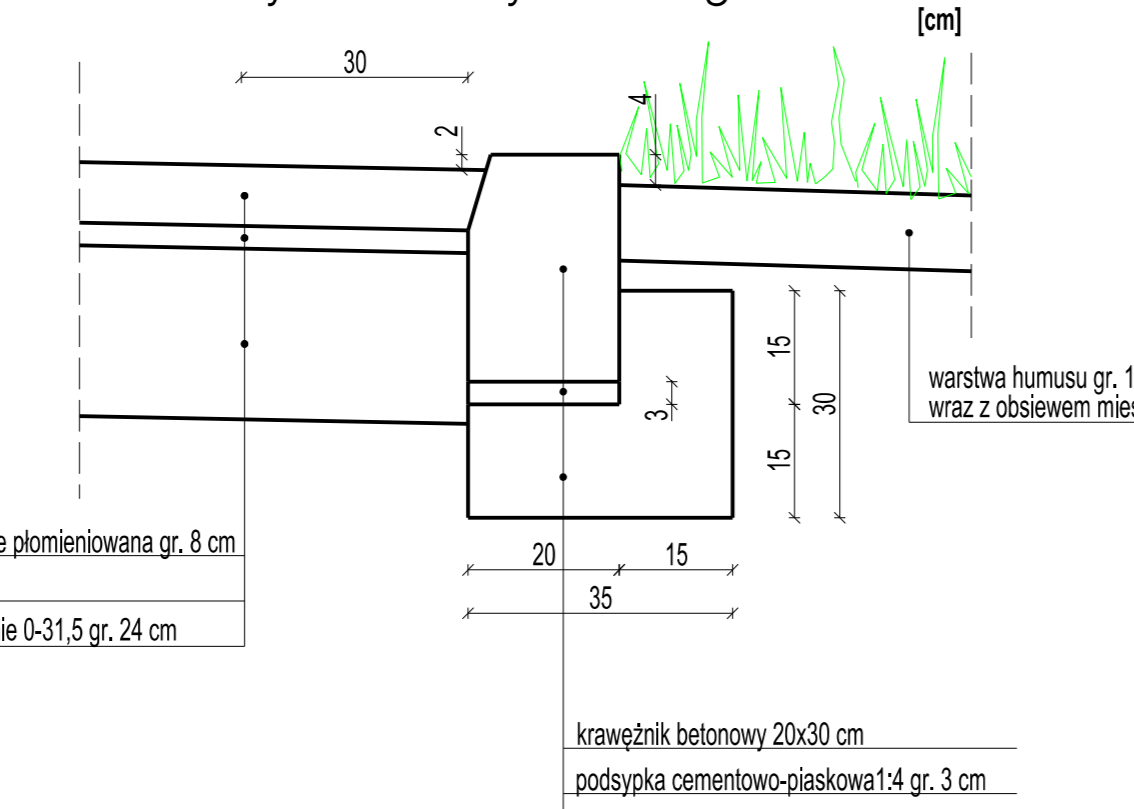
Szczegół krawędzi jezdni w obrębie skrzyżowania wyniesionego
