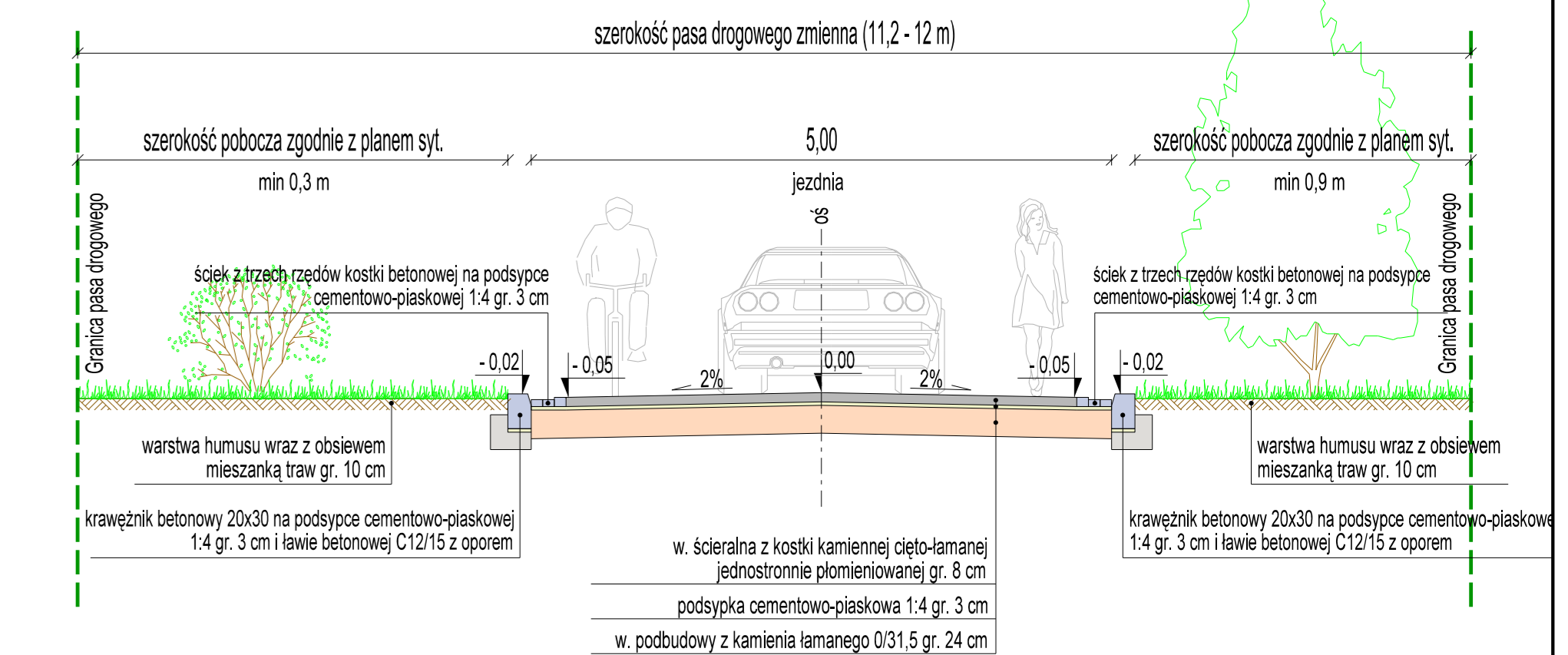
Przekrój normalny
