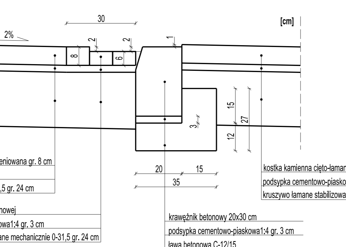
Szczegół połączenia zjazdu z jezdnią
