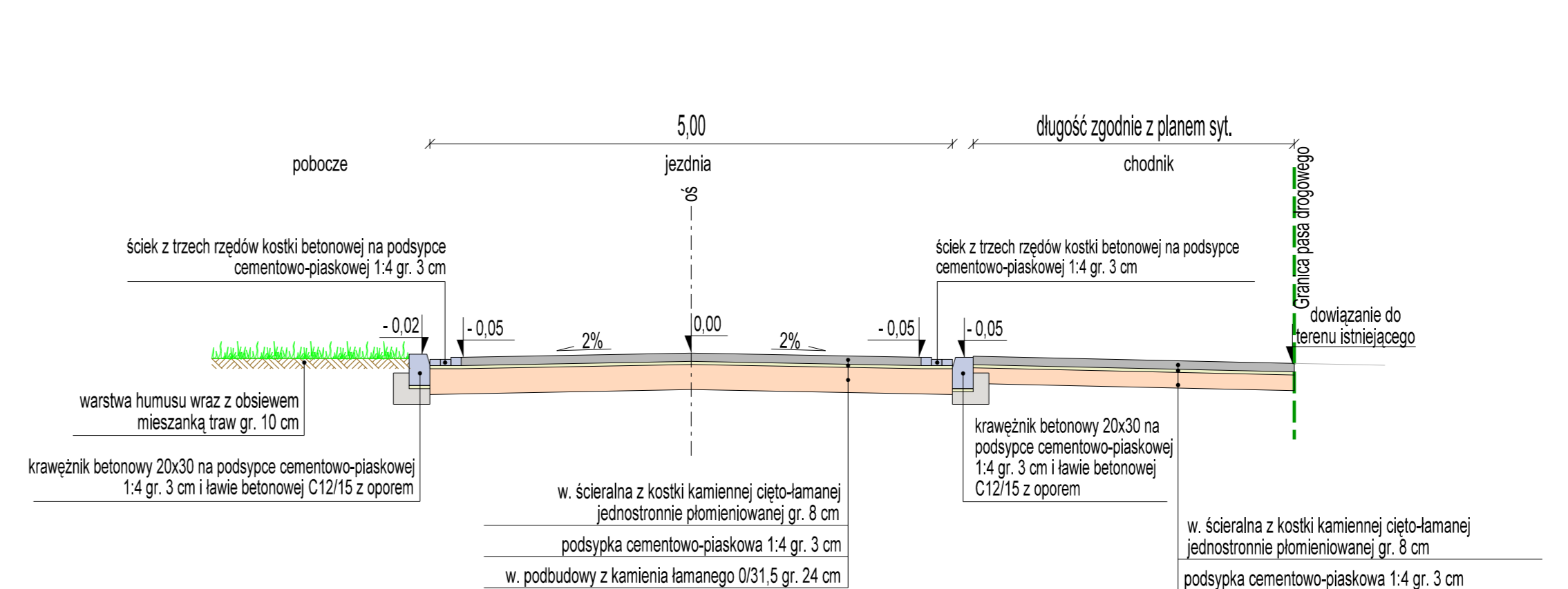
Przekrój przez chodnik do furtki
