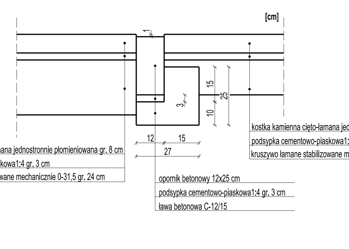
Szczegół połączenia zjazdu z chodnikiem
