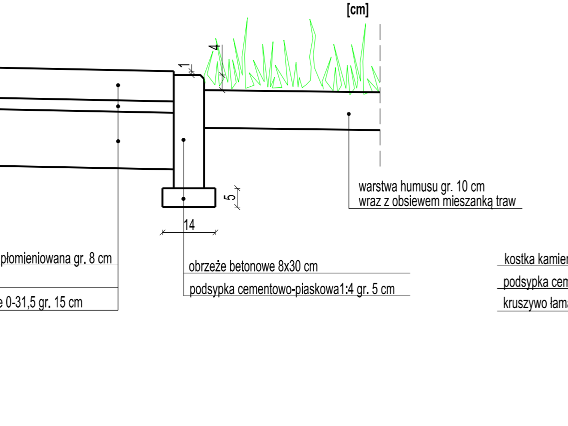
Szczegół krawędzi chodnika
