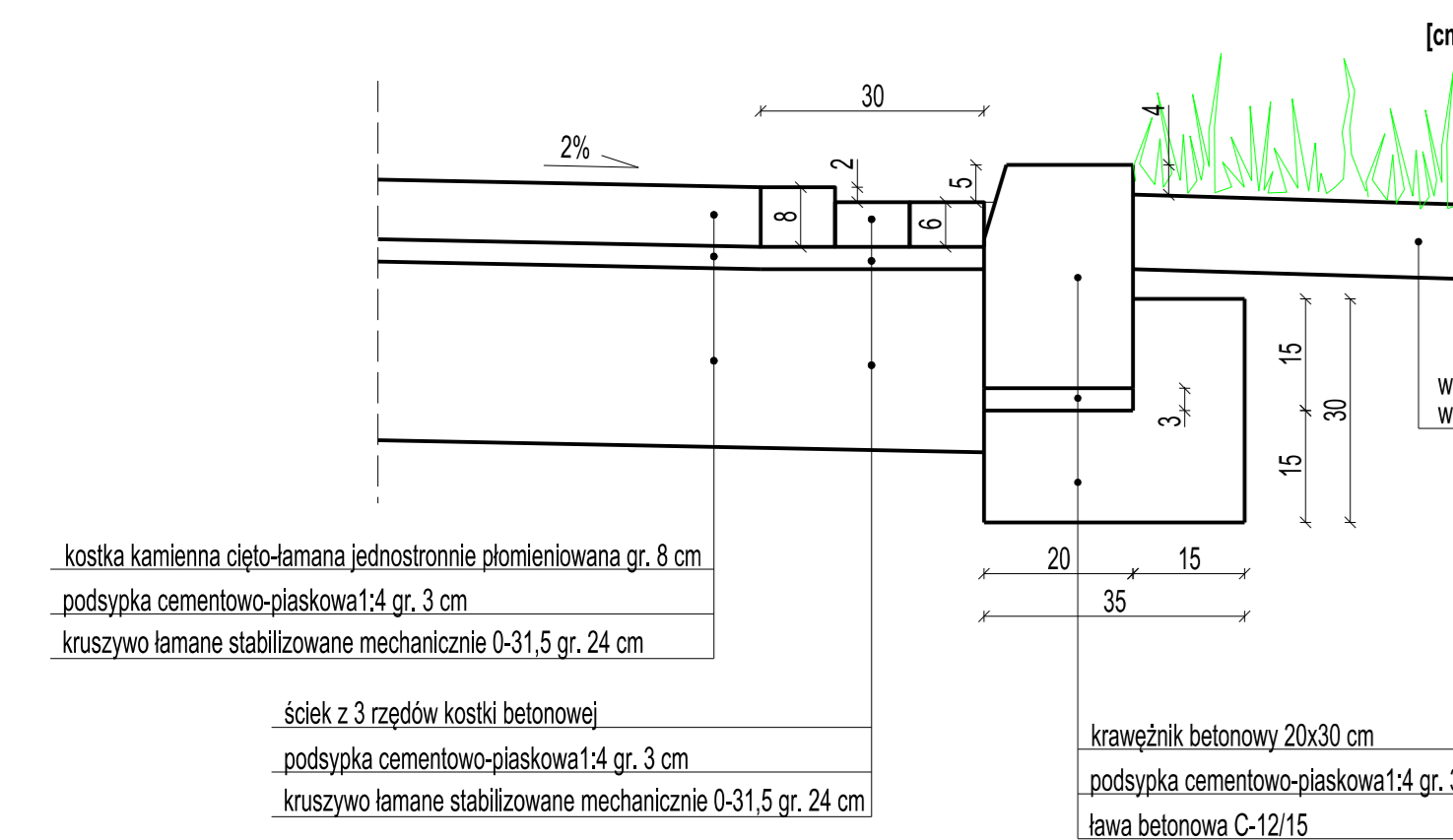
Szczegół ścieku przykrawężnikowego
