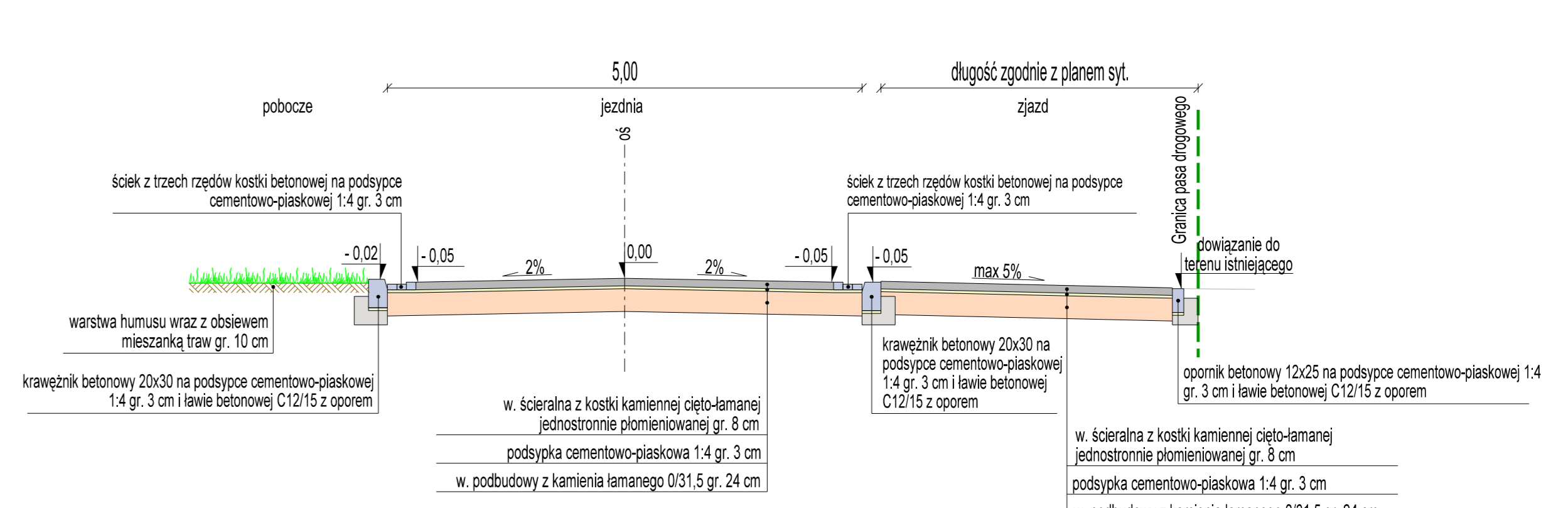
Przekrój przez zjazd
