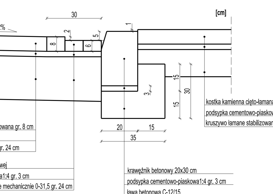
Szczegół połączenia chodnika z jezdnią
