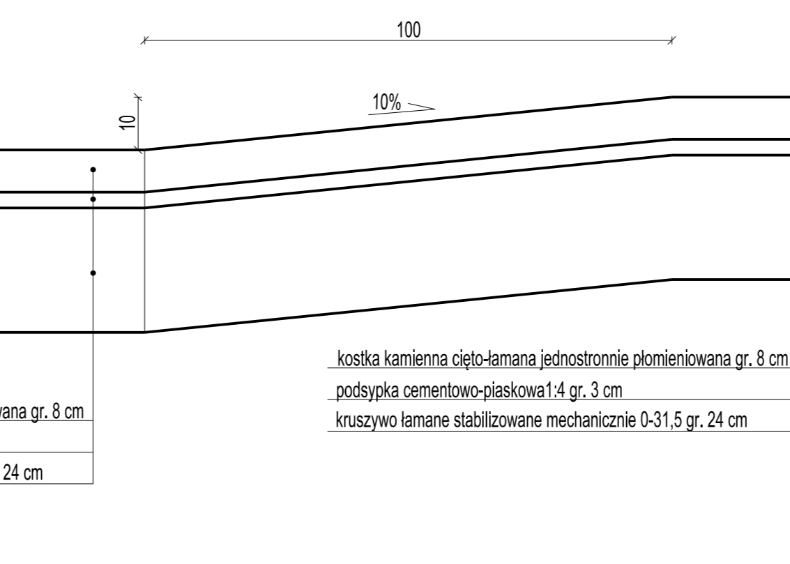
Szczegół rampy przed skrzyżowaniem wyniesionym
